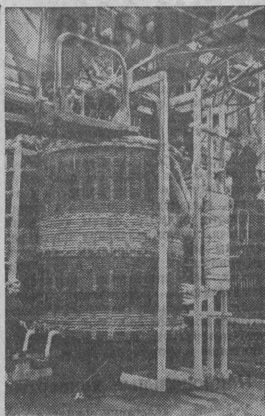
Коллектив московского трансформаторного завода имени Куйбышева собирает для Иркутской гидроэлектростанции мощную электрическую машину — автотрансформатор мощностью 188 тысяч киловольтампер на напряжении 220 тысяч вольт.
