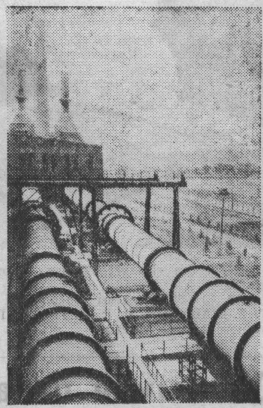
Грузинская ССР. Руставский цементный завод. Квартальный план выполнен успешно и дал несколько тысяч тонн цемента сверх плана. Недавно вступила в строй вторая очередь предприятия. На снимке: общий вид завода с двумя вращающимися печами. Фотохроника ТАСС.
