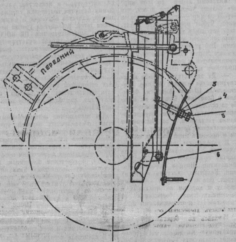
На рисунке: сошник с клапанным механизмом.
