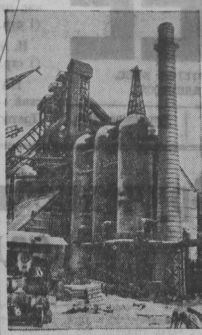
Вологодская область. В Директивах XX съезда КПСС по шестому пятилетнему плану намечено завершить строительство Череповецкого металлургического завода. НА СНИМКЕ: общий вид доменной печи № 2 Череповецкого металлургического завода. Фотохроника ТАСС.
