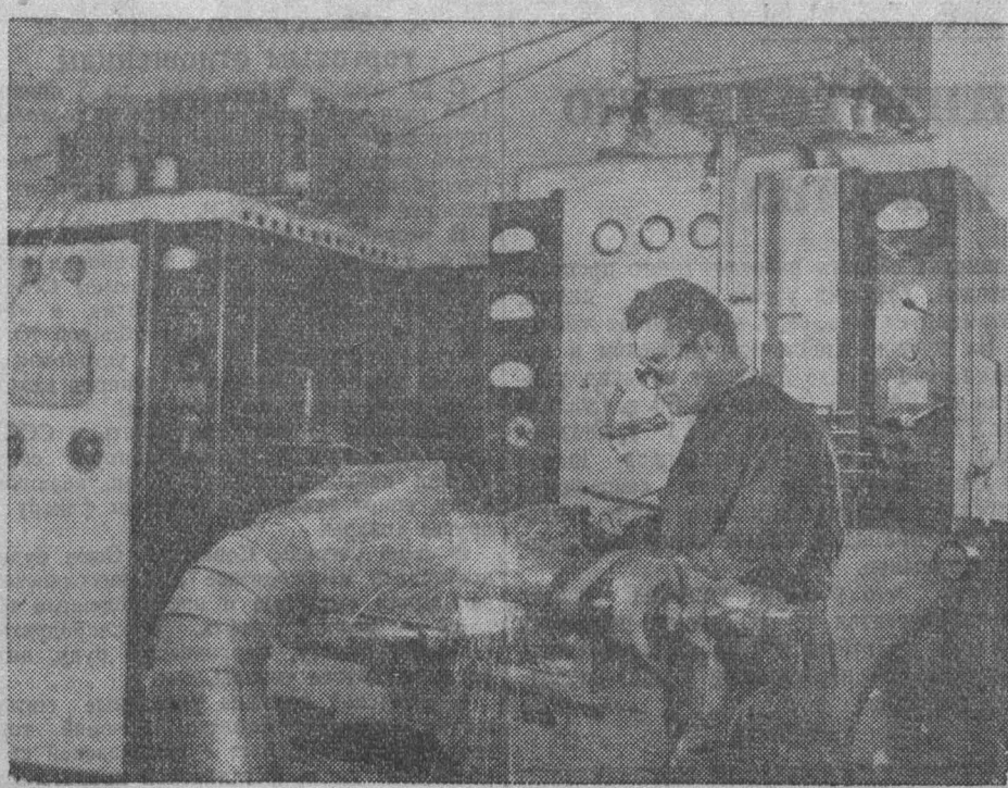
Запорожье. Научный сотрудник Запорожского филиала Всесоюзного научно-исследовательского института электрификации сельского хозяйства, кандидат технических наук К. П. Савинков с техником-электриком А. К. Козорезом разрабатывают новый способ металлизации деталей распылением металла с применением токов высокой частоты. Этот способ используется для восстановления деталей сельскохозяйственных машин. Он расширяет применение высокочастотных установок на ремонтных заводах Министерства сельского хозяйства: для поверхностной закалки, плавки металла, пайки, заливки биметаллических втулок (подшипников).
