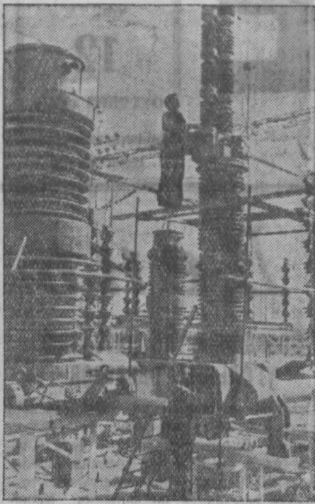
Московская область. В районе Ногинска заканчивается строительство подстанции, предназначенной для приема электроэнергии с Кубинской гидроэлектростанции. Первоначальное напряжение в 400,000 вольт здесь будет понижаться до 220,000 и 110,000 вольт. НА СНИМКЕ: бригадир И. Ф. ГРИШЕНКО (вверху) и слесарь-механик В. В. КОРЧУКОВ за наладкой воздушных выключателей. Фотокроника ТАСС.
