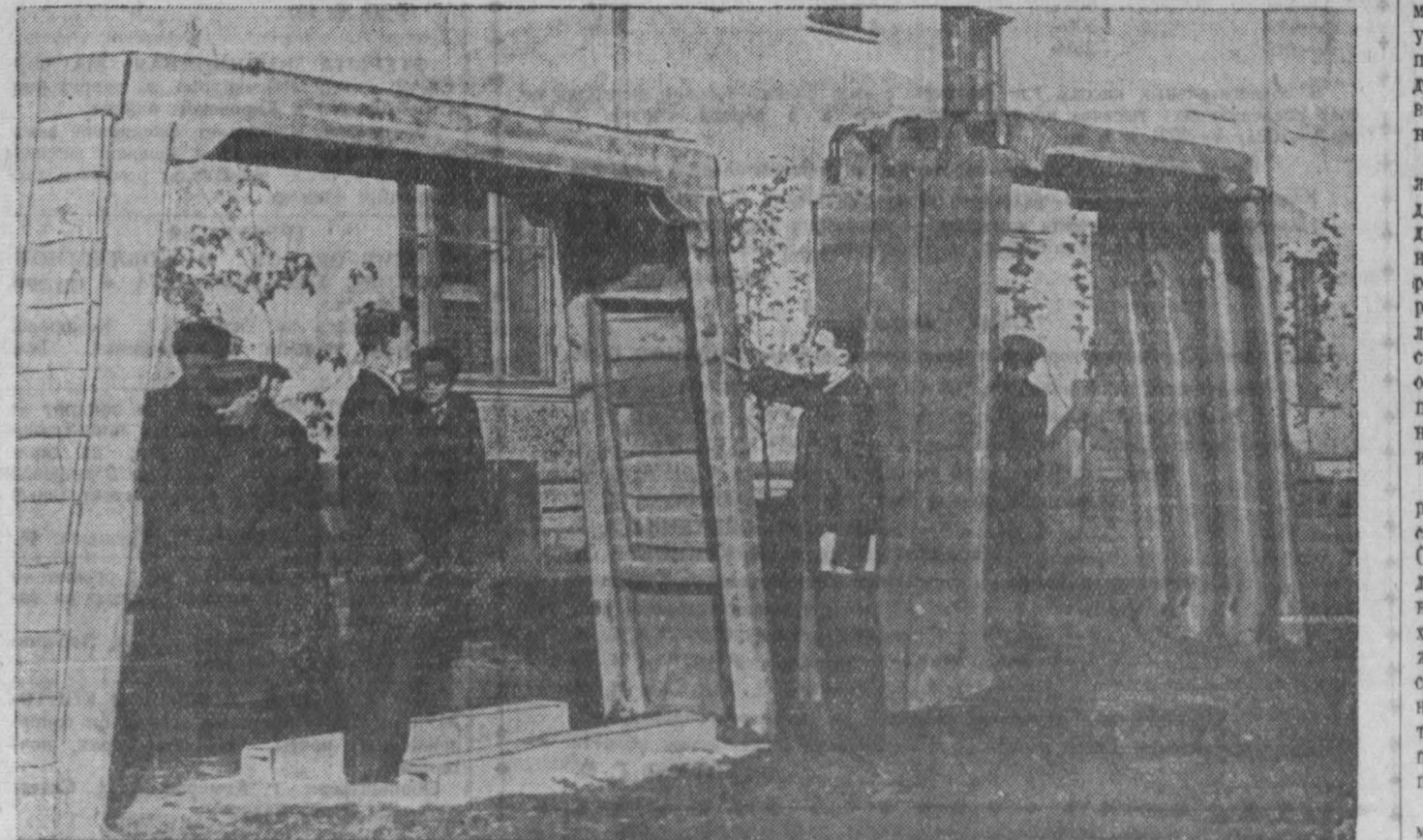
В залах Дома техники комбината «Кузбассшахтострой» и на прилегающей к нему территории в дни работы совещания была организована строительная выставка. На ней представлены разнообразные конструкции и детали из сборного железобетона, выпуск которых освоен или осваивается на заводах и полигонах комбината. НА СНИМКЕ: группа участников совещания знакомится со сборным железобетонным креплением для горизонтальных гор- Фото В. Булечева.
