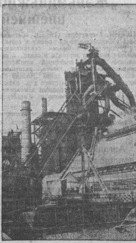
Ворошиловградская область. На металлургическом заводе имени Ворошилова недалеко слана в эксплуатацию новая доменная печь, рассчитанная на повышенное давление газа под колосников и оборудованная новейшей отечественной аппаратурой с автоматическим управлением.
