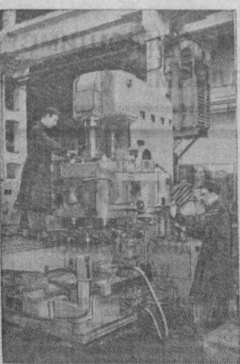
На московском заводе «Станкоконструкция» изготовлена партия човых копировально-фрезерных станков-полуавтоматов. На них можно обрабатывать одновременно две детали самой сложной конфигурации с точностью до 0,05 миллиметра. Станок управляется посредством сложной гидравлической системы. Копировально-фрезерный полуавтомат позволяет повысить производительность труда в восемь-десять раз.
