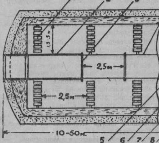
Рис. 4. План бурта. 1. Приточные каналы, проходящие под продукцией. 2. Стойки. 3. Распоры. 4. Прогоны. 5. Треугольные щиты. 6. Стенки тамбура. 7. Решетчатая дверь. 8. Наружная дверь.
