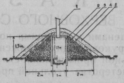
Рис. 1. Бурт с картофелем. 1. Вытяжная труба. 2. Стенки коридора. 3. Картофель. 4. Солома. 5. Земля.
