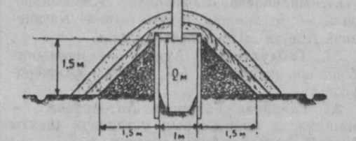
Рис. 2. Бурт с капустой.
