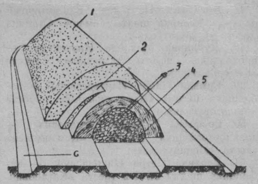
Рис. 5. Бурт с гребневой вентиляцией. 1. Полная зимняя крышка. 2. Предварительная земляная крышка. 3. Контрольная трубка для измерения температуры. 4. Солома. 5. Картофель. 6. Водосточный канал.
