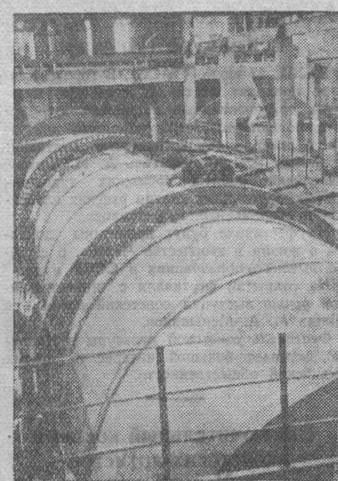
Киевская область. На окраине Мирановки, Старченковского района, выстроился корпус нового крупного предприятия. Это — один из пяти строящихся на Украине сахарных заводов. В этом году он вступит в строй. Завод оснащается новейшей техникой. НА СНИМКЕ: монтаж непрерывно действующего диффузионного аппарата. Фототехника ТАСС.
