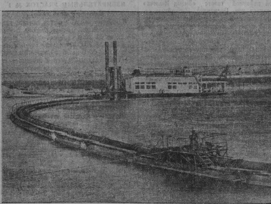
«Сталинградгидрострой». Сверхмощный земснаряд «Сталинградский-1005» производит выемку грунта из котлована под водосливную плотину.
