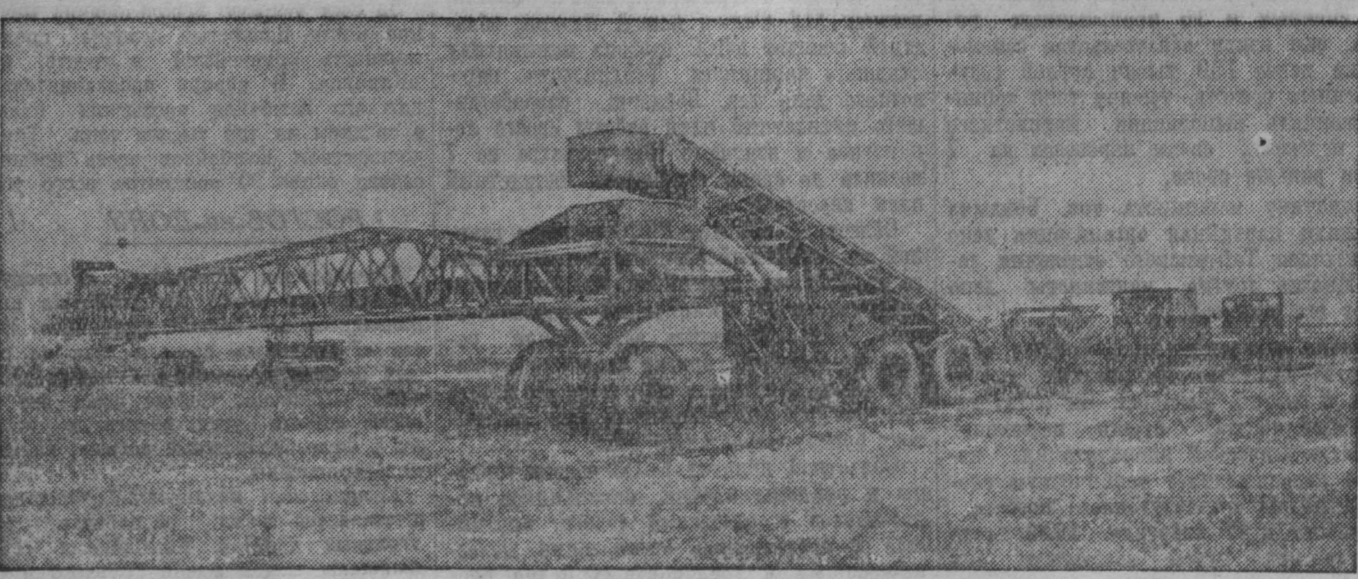
Парк разнообразных машин и механизмов действующих на строительных площадках гигантских гидроузлов и каналов, непрерывно пополняется техникой новых образцов. НА СНИМКЕ: новая мощная машина — землеройный строг «Д-26», предназначенный для работы на строительстве судоходных и крупных магистральных оросительных каналов.
