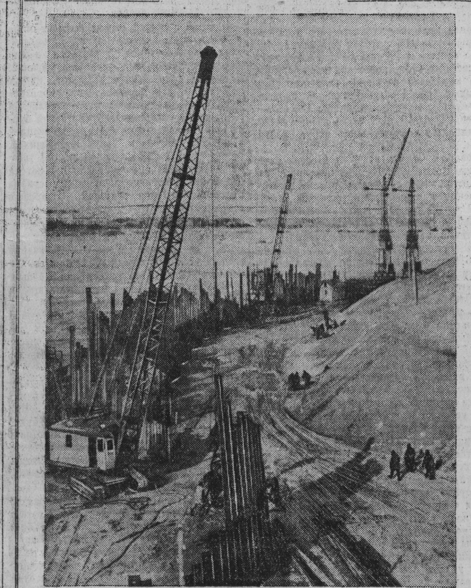
Сталинградгидрострой. Строительство великого сооружения у стен Сталинграда принимает все более широкий размах. НА СНИМКЕ: строительство шпунтовой перемычки на левом берегу Волги, ограждающей котлован, где будет сооружаться здание Сталинградской ГЭС. Фотохроника ТАСС.
