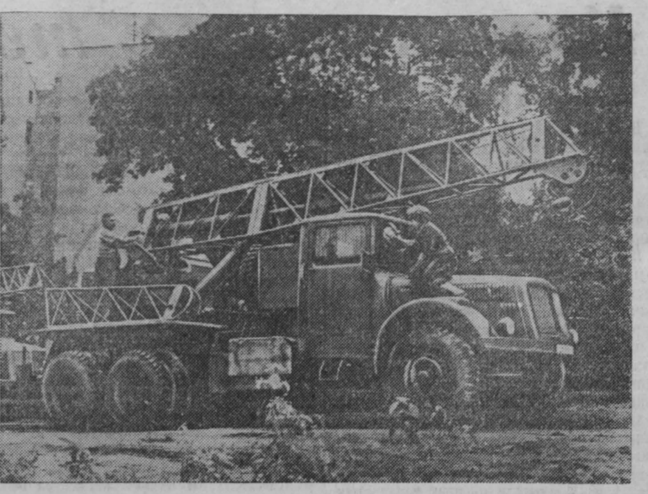
Чехословацкая Республика. Коллектив машиностроительного завода имени Швермы в Праге-Височаны закончил монтаж нескольких передвижных подъемных вращающихся кранов на автомобильном ходу.
