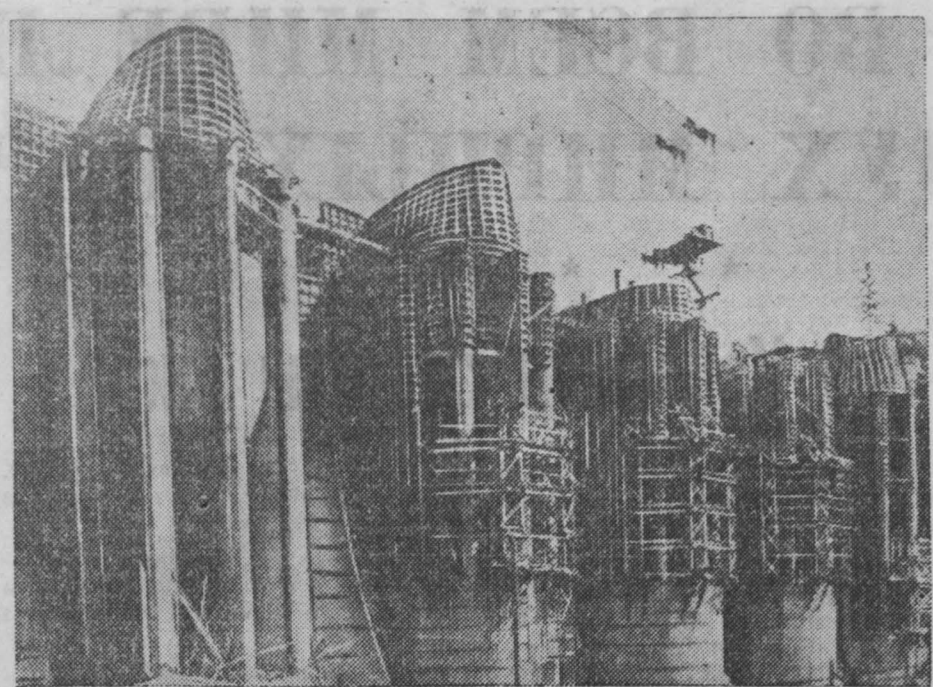
Чехословацкая республика. Строительство Слупской плотины в Средней Чехии. Высота плотины—70 метров. Она образует водохранилище длиной в 44 километра. По другую сторону плотины строится мощная гидроэлектростанция. НА СНИМКЕ: общий вид строящейся Слупской плотины. Фото Чехословацкого телеграфного агентства.
