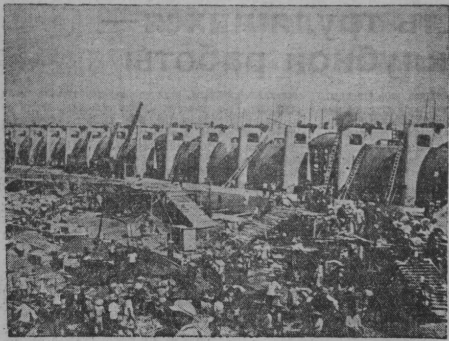
Народное правительство Китая успешно осуществило огромные ирригационные работы. Эти работы обеспечивают им высокие урожаи. НА СНИМКЕ: строительство плотины в среднем течении реки Янцзы. Фото агентства Синьхуа.
