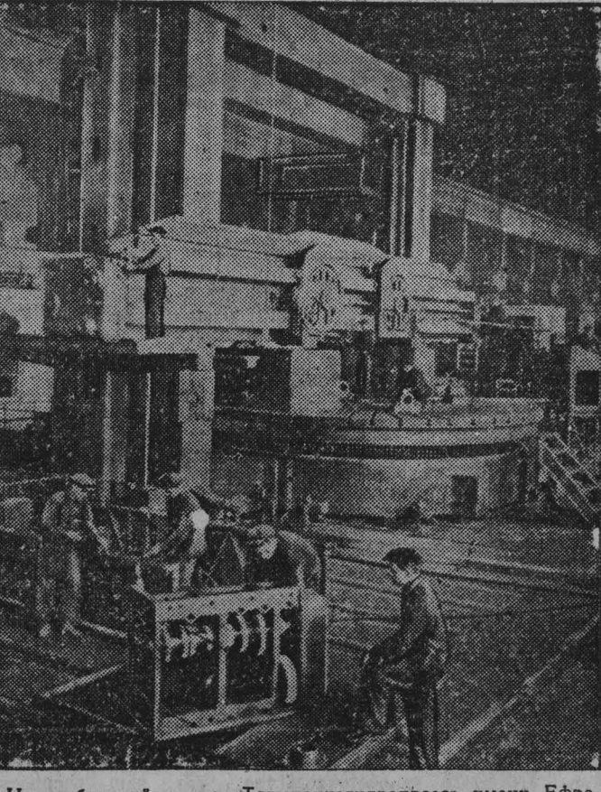
Новосибирский завод «Тяжстанкогидропресс» имени Ефремова выпускает новые типы уникальных станков. Независимо закончена сборка мощного карусельного станка, на котором будут обрабатываться детали турбин и других агрегатов для великих строек коммунизма. Размеры станка позволяют обрабатывать детали, размером более семи метров и весом до ста шестидесяти тонн.
