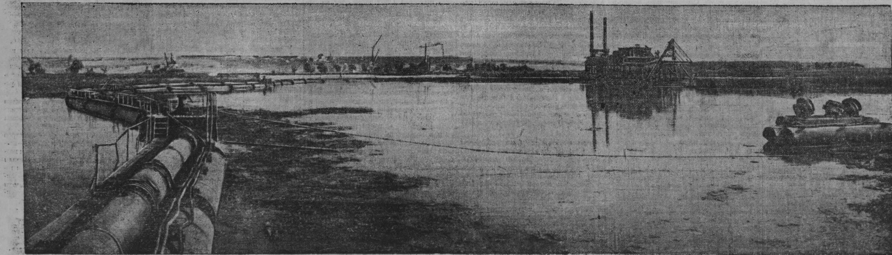
Новая Каховка. Все шире развертывается строительство Каховского гидроузла. С полной нагрузкой работают земснаряды на сооружении котлована водосливной плотины и шлюза. Производственная мощность земснарядов, работающих в Днепровской пойме, составляет 35 тысяч кубометров грунта в час. НА СНИМКЕ: земснаряд за работой.
