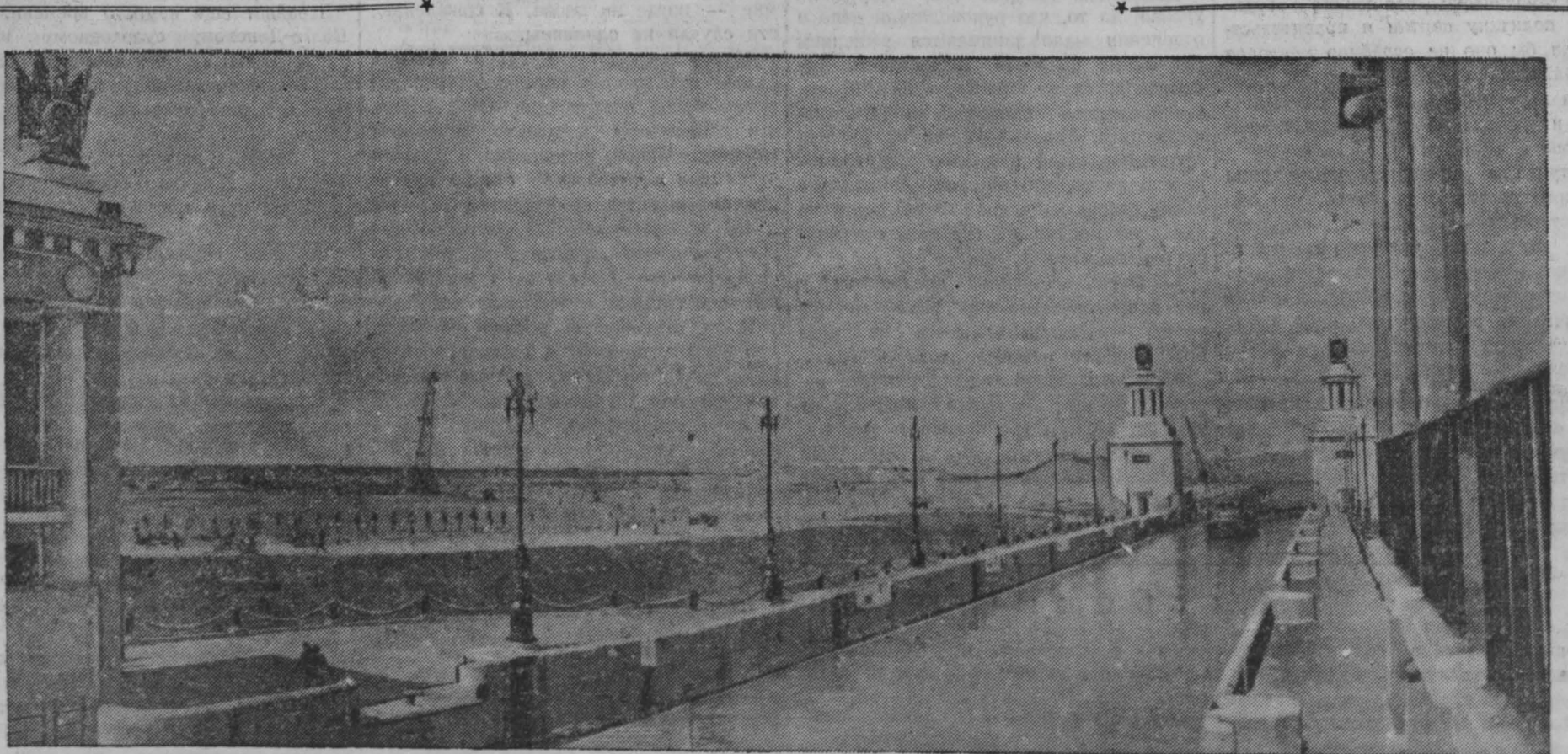
ВОЛГО-ДОНСКОЙ СУДОХОДНЫЙ КАНАЛ ИМЕНИ В. И. ЛЕНИНА. НА СНИМКЕ: общий вид заполненной водой камеры 9-го шлюза в момент входа в нее судов.
