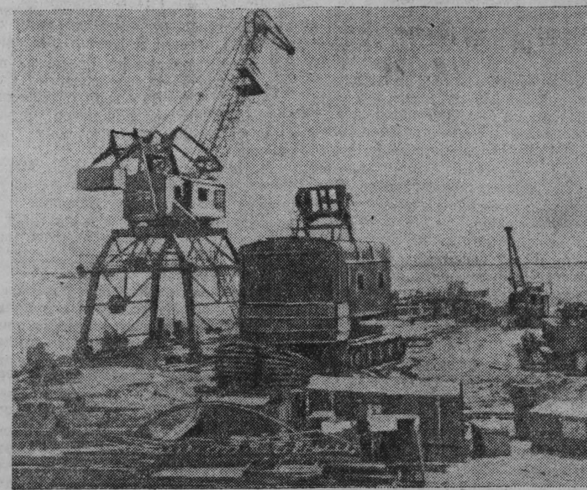
ТАХИА-ТАШ. На монтажной площадке в Тахиа-Таше заканчивается сборка семикубового электрического экскаватора.
