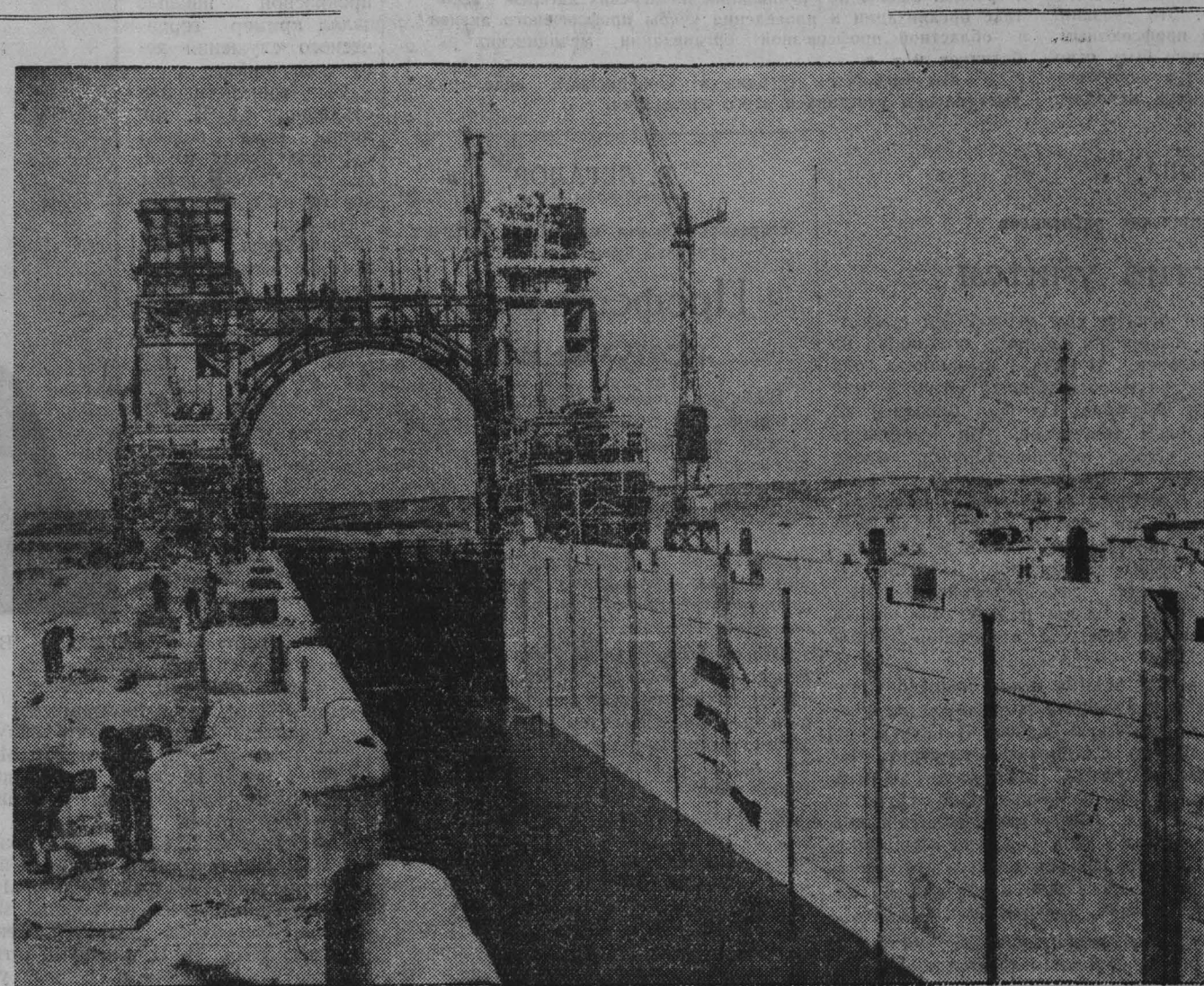
ВОЛГОДОНСТРОЙ. Камера 13-го шлюза, заполненная донской водой.
