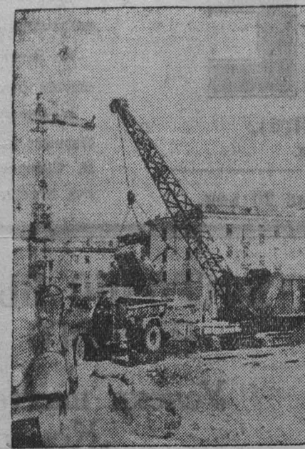
Г. Кемерово благоустраивается. Экскаватор производит выемку грунта по Кузнецкой улице. Фото П. Косюкова.
