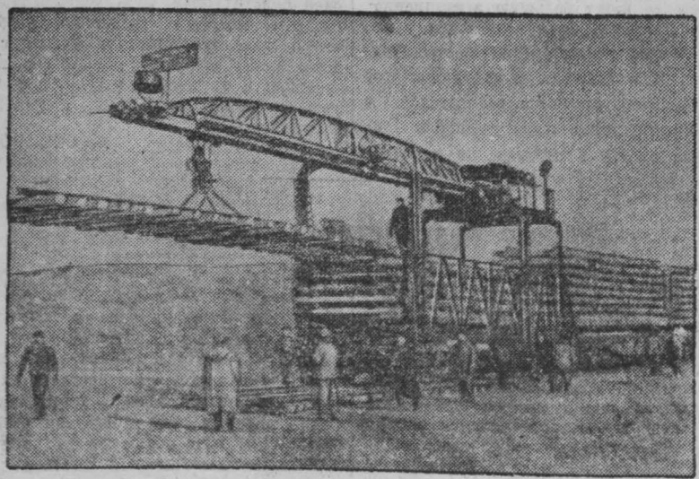
КУБЫШЕВГИДРОСТРОЙ. Бригада дорожного мастера Ф. Е. Садкова на строительстве железнодорожного подвального пути укладывает при помощи путеукладчика системы Платова по одному километру пути в смену.
