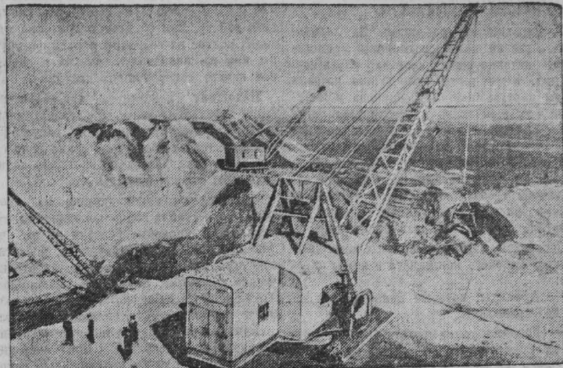
Шагающий экскаватор в одном из карьеров Бачатского угольного разреза. (Фотохроника ТАСС).
