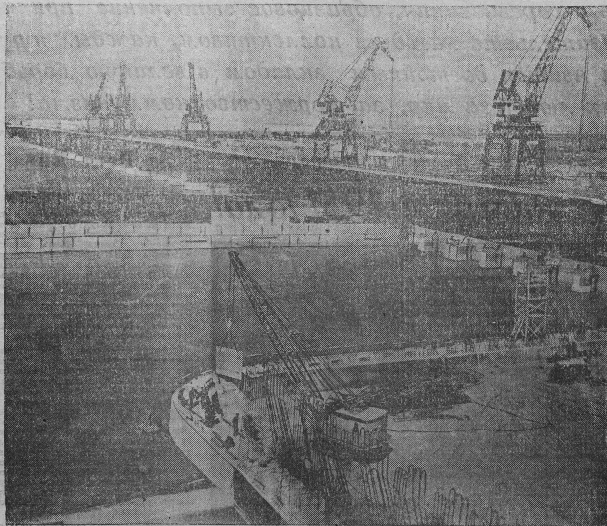
НА СТРОИТЕЛЬСТВЕ ДНІПРОВСЬКОГО ГІДРОУЗЛА. Дон пошел по новому руслу через гидротехнические сооружения. НА СНИМКЕ: общий вид котлована, затопленного водами Дона. (Фотохроника ТАСС).
