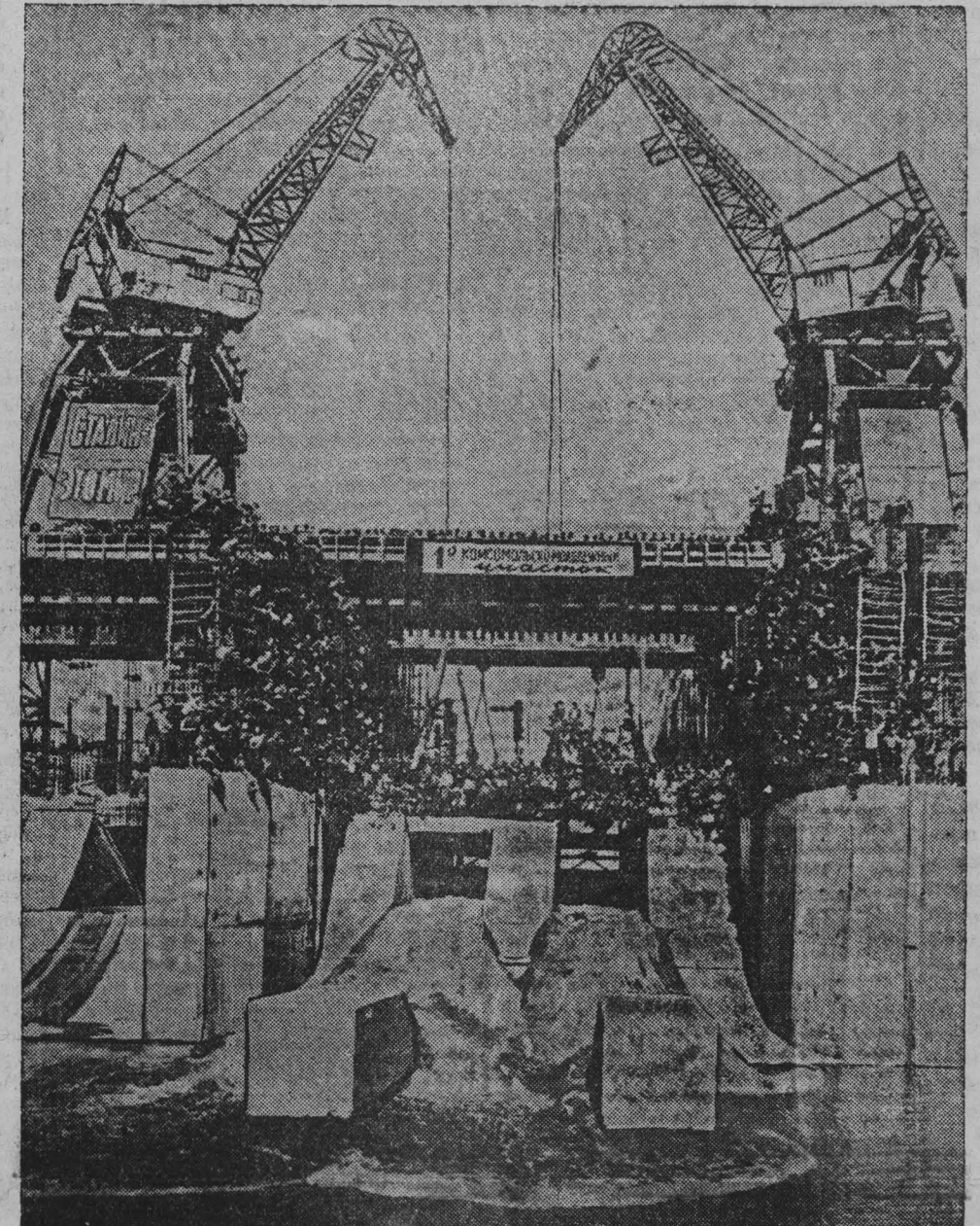
На строительстве Цимлянского гидроузла 20 сентября 1951 года. НА СНИМКЕ: момент поднятия заслонок первых двух допных ответвений в основании водосливной плотины и пуска вод Дона через водосливную плотину Цимлянской ГЭС.
