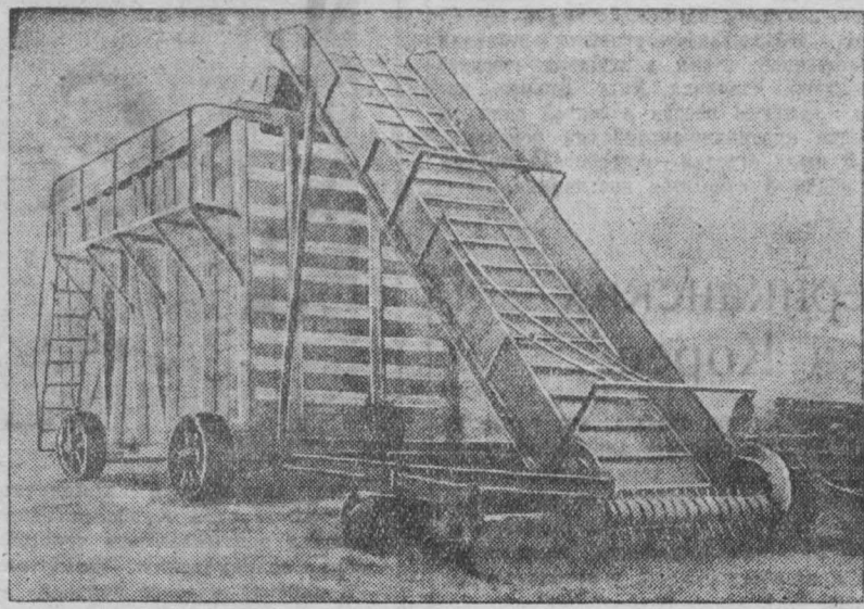
Подборщик-стогомет.
