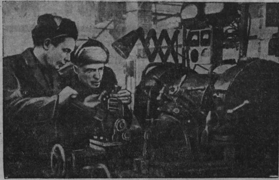
На Кузнецком машиностроительном заводе сейчас заканчиваются испытания анодно-механического станка для заточки буровых коронок. Благодаря точной обработке стойкость коронок, заточенных на этом станке, увеличивается в несколько раз. На этом станке можно будет обрабатывать любые коронки. На снимке: старший мастер Ф. Кудрявцев и технолог Я. Верник за испытанием станка. Снимок В. Бульчева.
