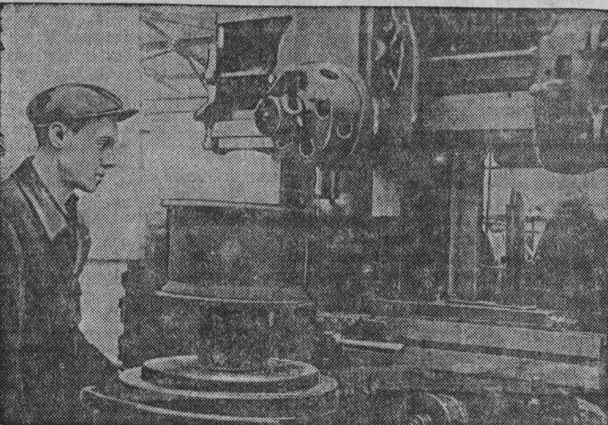
Токарь-карусельщик В. А. Тарасов руководит одной из лучших комсомольско-молодежных бригад Кемеровского электромеханического завода. Сам бригадир за четыре послевоенных года выполнил 7 годовых норм. На снимке: В. А. Тарасов за работой. Снимок И. Иванова.
