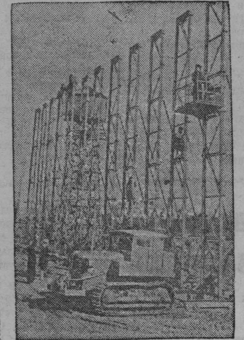
Новосибирск. Заводу строительных машин поручено изготовить для строительства Куйбышевской гидроэлектростанции партию мачтовых подьемников. Коллектив предприятия с большим воодушевлением принялся за выполнение почетного заказа. Сейчас заканчивается монтаж первой партии подьемников, которые будут отправлены в адрес «Куйбышевгидростроя».
