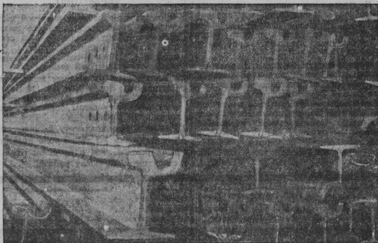
Рельсы «Феникс», прокатанные на Кузнецком комбинате для Московского метро и трамвая. Фото. В. Бульчева.
