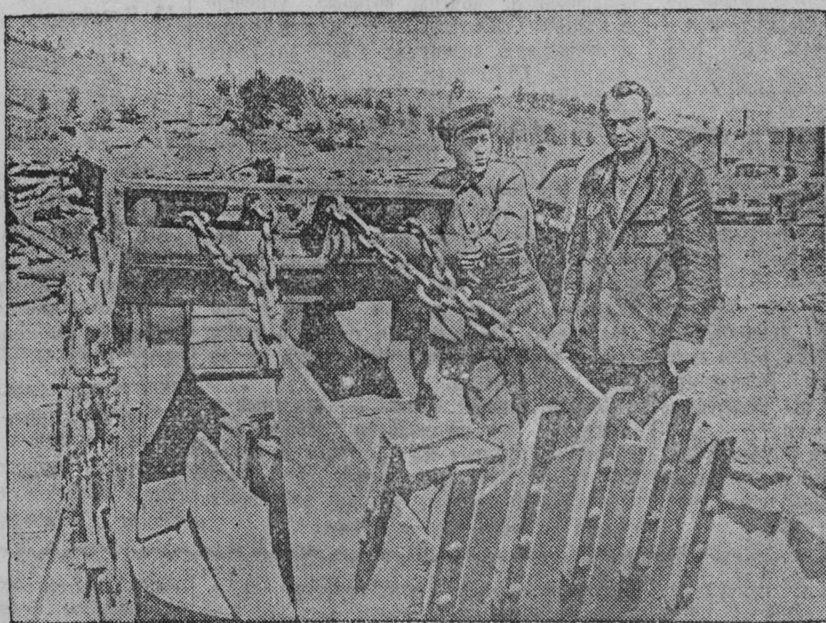
Шахта «Ахашево-2», вступившая в строй в 1948 году, является одной из наиболее механизированных шахт Кузбасса. Она непрерывно пополняется новейшими машинами. На снимке: прибыла новая углепогрузочная машина.
