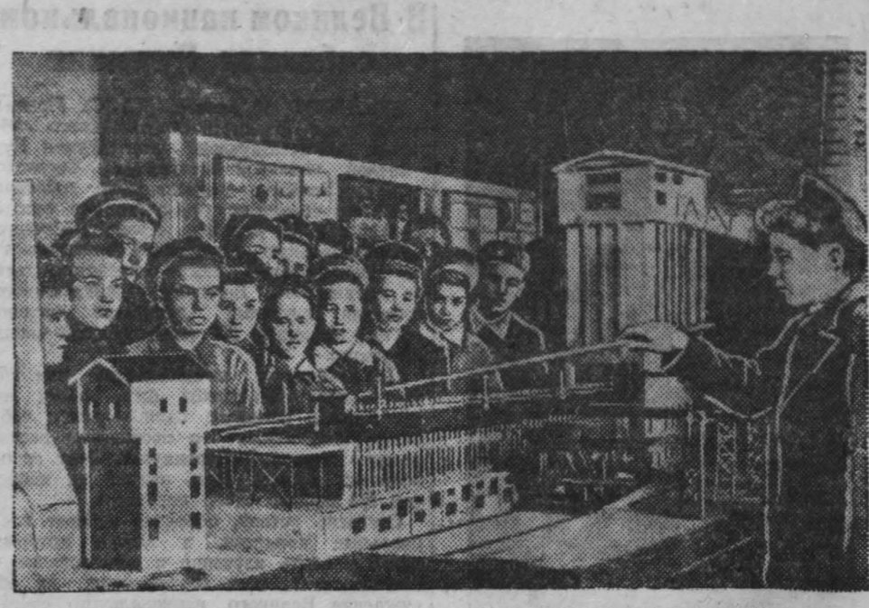
Дому техники Кузнецкого металлургического комбината исполнилось 15 лет. На снимке: инженер-экскурсовод тов. А. Д. Амеулова в коковом отделе Дома техники объясняет группе учащихся ремесленного училища устройство коковской печи. Фото В. Булмачева.
