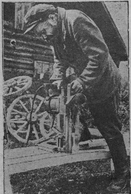
Свердловская область. В колхозе «Пролетарка», Красносельского района, электрифицированы мастерские по ремонту и изготовлению сельскохозяйственного инвентаря. На снимке: колхозный столяр Я. З. Теменов работает на электродолбежном станке.
