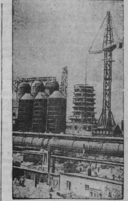
Зaporozhye. Заключается строительство доменной печи № 4 завода «Запорожсталь». Это будет первая в СССР цельносварная доменная печь.
