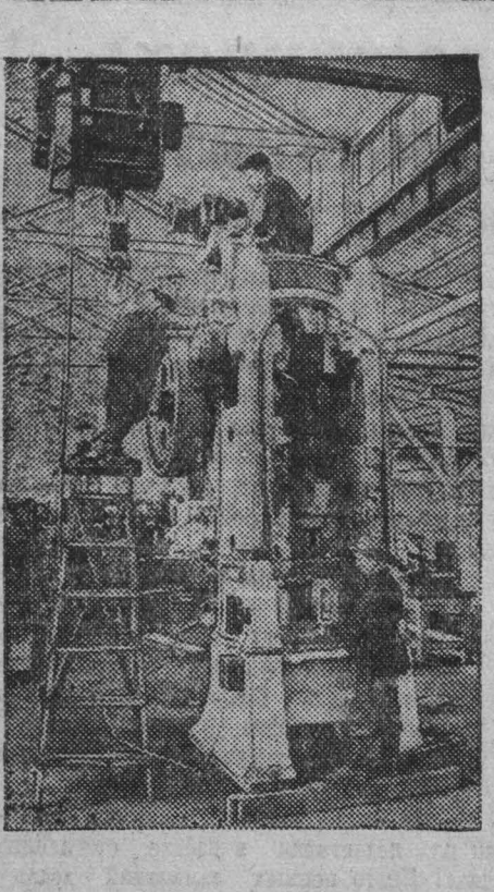
Алтайский край. Барнаульский завод механических прессов освоил производство мощных 150-тонных прессов. На снимке: монтаж пресса в сборочном цехе.
