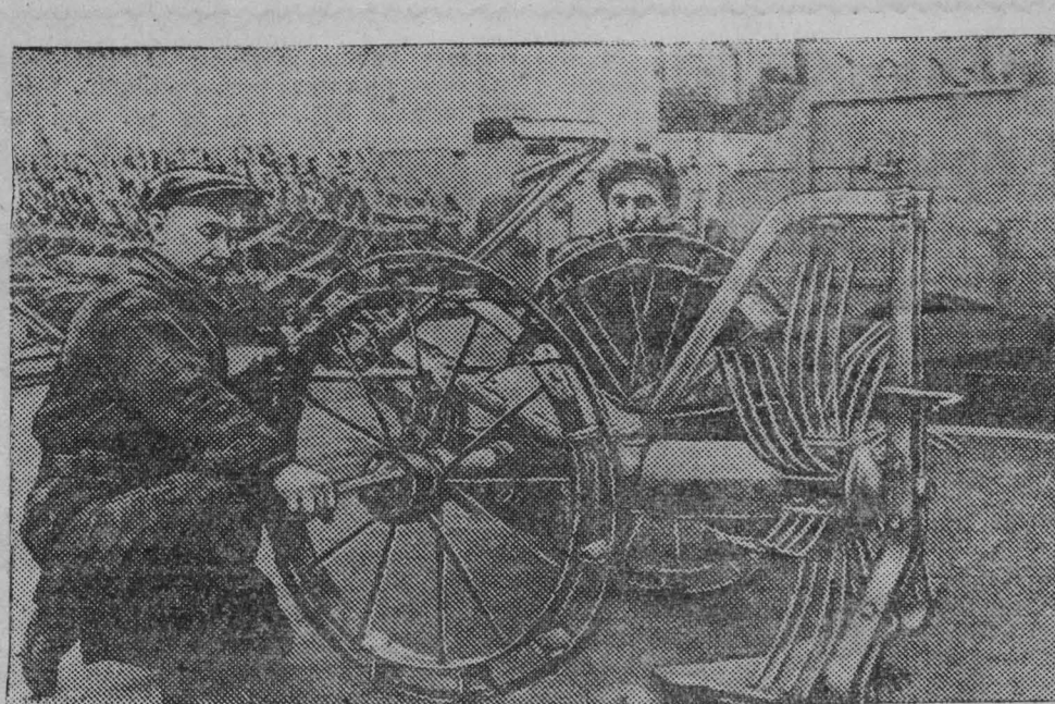
Таллин. Завод сельскохозяйственных машин Союза потребительских обществ (ЭТКВД) освоил производство картофелекопалок. В этом году завод изготовит тысячи таких машин. На снимке: в сборочном цехе завода. Слева Р. Тиннас (слева) и О. Варму за сборкой картофелекопалки. (Фотохроника ТАСС).
