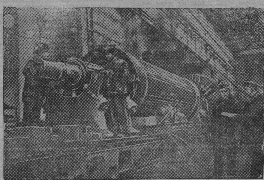
Ново-Краматорский ордена Ленина машиностроительный завод имени Сталина (Донецк). На снимке: обработка и проверка ротора турбины для Зуевской электростанции. (Фотохроника ТАСС).
