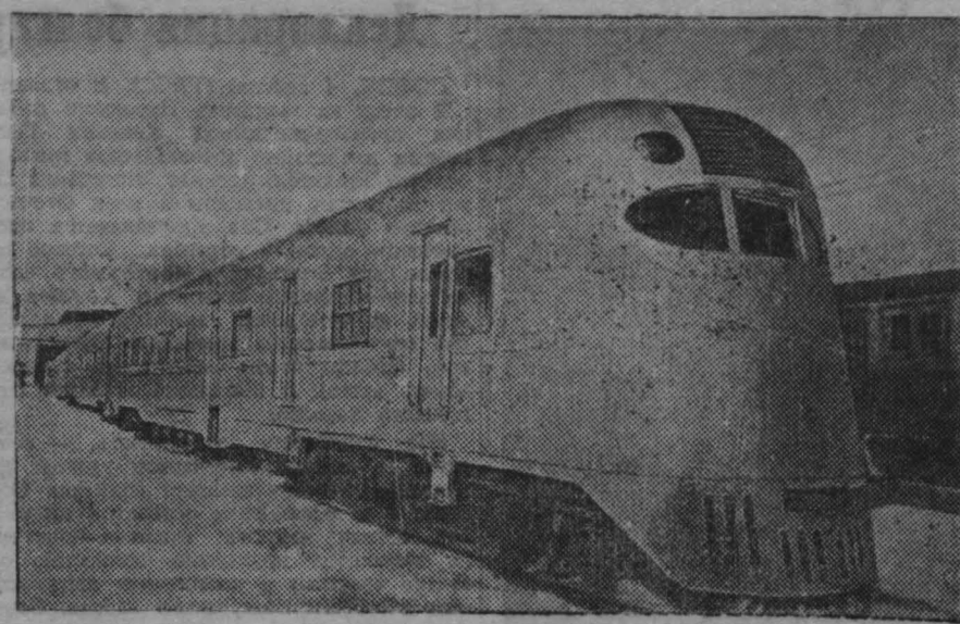
В ближайшее время в Москву прибывает новый скоростной дизельный поезд. Он приводится в движение двумя дизельными моторами по 310 лошадиных сил, расположенными в обоих концах состава. Вагоны, рассчитанные на 156 пассажиров, комфортабельно оборудованы. Несколько таких поездов скоро начнет курсировать на железных дорогах страны.
