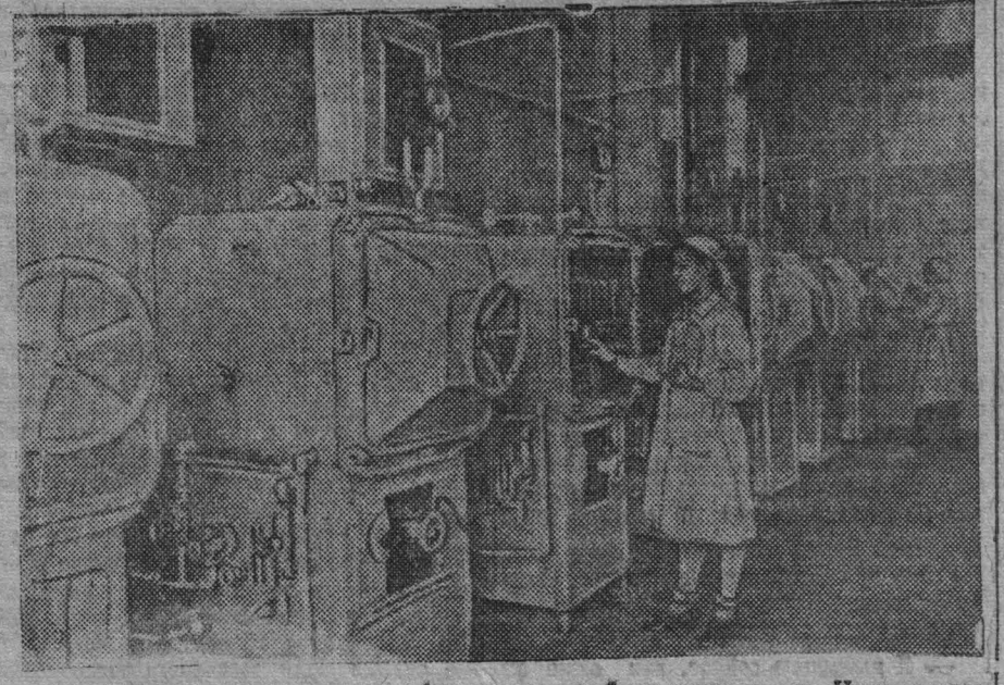
На Московском заводе химико-фармацевтической промышленности Наркомздрава СССР сданы в эксплуатацию крупнейший в Союзе цех по производству пенициллина. В трех этажах большого заводского корпуса установлены сложные аппараты и механизмы для получения препарата. На снимке: стерилизация питательных сред в автоклавах. (Фотохроника ТАСС).
