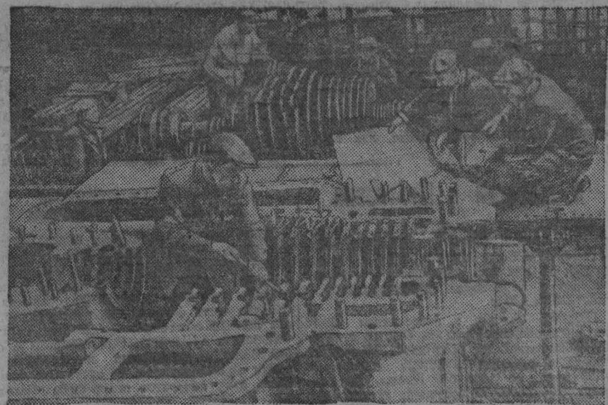
Коллектив турбинного пеха Кировского завода (Ленинград) восстанавливает для металлургического завода Кривоножко паровую турбину мощностью в 12 тысяч киловатт.
