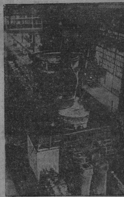
Кузнецкий металлургический комбинат. Разливка стали через промежуточное устройство. Фото А. Фатеева.
