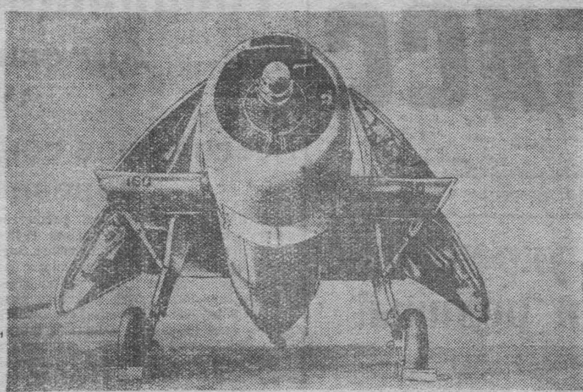
На снимке: американский самолет-торпедоносец «Эванджер», применяемый для нападения на неприятельские торговые суда. Крылья самолета складываются при помощи гидравлического механизма и под дном его помещается торпеда, весящая около 900 килограммов.
