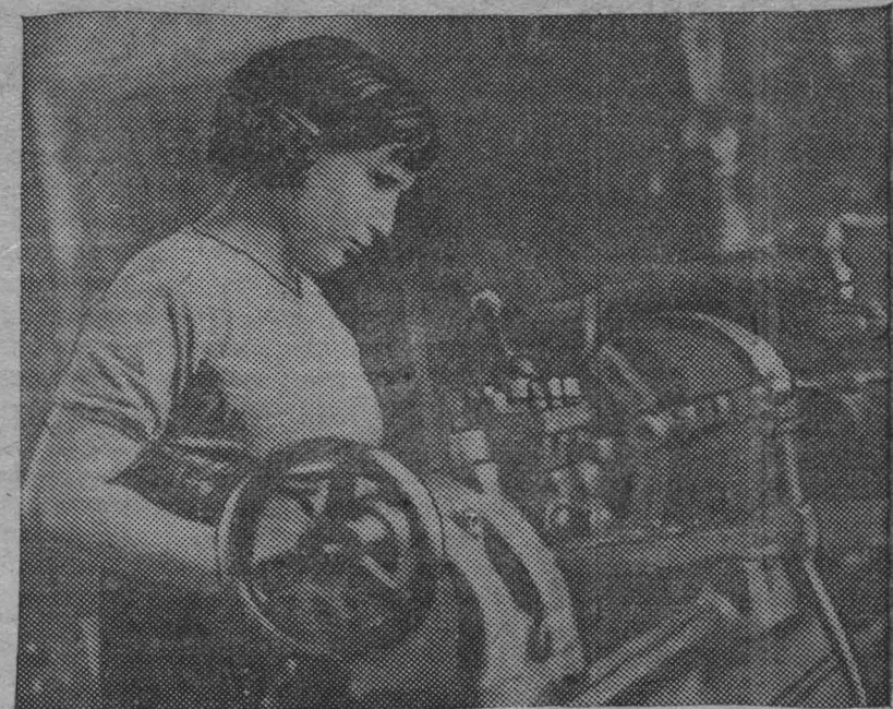
Инструментальщина железнодорожного депо ст. Кемерово тов. А. Чалпанов успешно изучил токарное дело и выдержал испытание на хорошо. Теперь она работает самостоятельно. На снимке: тов. Чалпанов за отточкой американского соединения для вагонов. Фото Толстикова.
