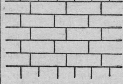
Американская кладка.
