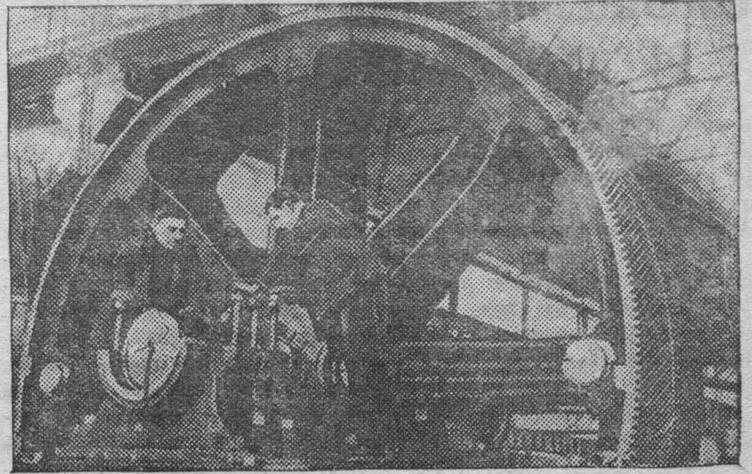
На Краматорском машиностроительном заводе им. Сталина монтажная бригада мастера тов. Осипова заканчивает изготовление шахтного подъемника, диаметр барабана которого равен 5 метрам.
