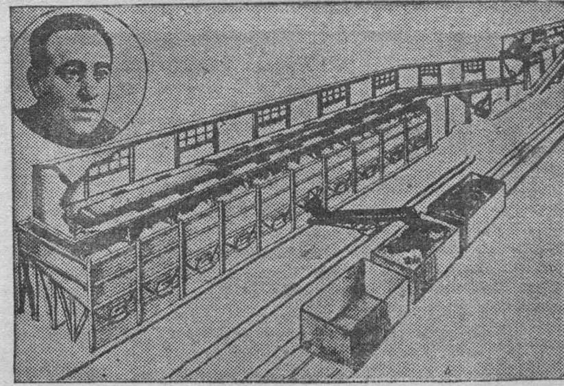
Инструктор-механизатор И. М. Розенвассер применил на шахтах Донбасса методы тов. Блиамина для погрузки угля из под эстакад в железнодорожные вагоны. Комплексно-механизированная погрузка угля по схеме тов. Розенвассера, примененная на шахтах 8 Чулюкка и 9 Наклонная (Донбасс) резко увеличила производительность труда. На снимке: Схема комплексно-механизированной погрузки угля на шахте 8 Чулюкка. В овале — И. М. Розенвассер. Фотохроника ТАСС.
