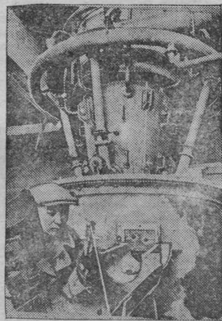
На Кольском полуострове у подножья гор Мончо-Тундры строится мощный Северный никелевый комбинат. На снимке: Ватержетная печь для плавки богатых жильных руд в металлургическом цехе опытного завода „Североникеля“.
