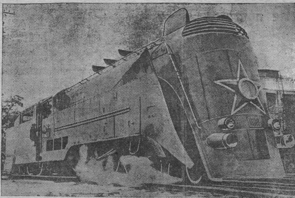
Коломенский машиностроительный завод им. В. В. Куйбышева выпустил второй скоростной паровоз „2-3-2“. После заводских испытаний паровоз испытывается на Октябрьской железной дороге. На снимке: Паровоз „2-3-2“. Союзфото.
