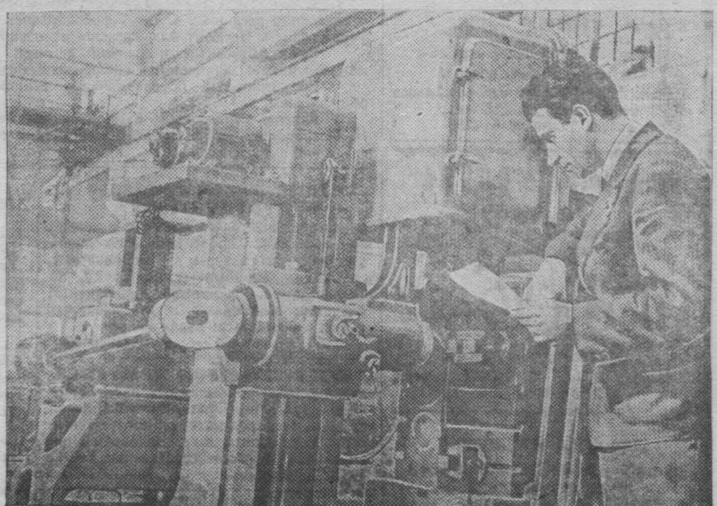
Станок, читающий чертёжи. Аспирант Московского станко-инструментального института инженер-механик В. С. Вихман изобрел фото-электрический металлообрабатывающий фрезерный станок, производящий обработку сложных фасонных деталей автоматически по чертежу, вложенному в станок. В Центральном Научно-исследовательском институте машиностроения построен первый опытный промышленный экземпляр нового станка. Станок В. С. Вихмана значительно ускоряет время изготовления сложных деталей и повышает точность. НА СНИМКЕ: изобретатель инженер В. С. Вихман у изобретенного им станка. Союзфот.
